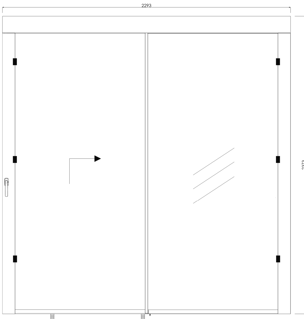
Fig. 1. Prospetto del campione sottoposto a prova_vista interna (dimensioni nominali dichiarate, espresse in mm)
