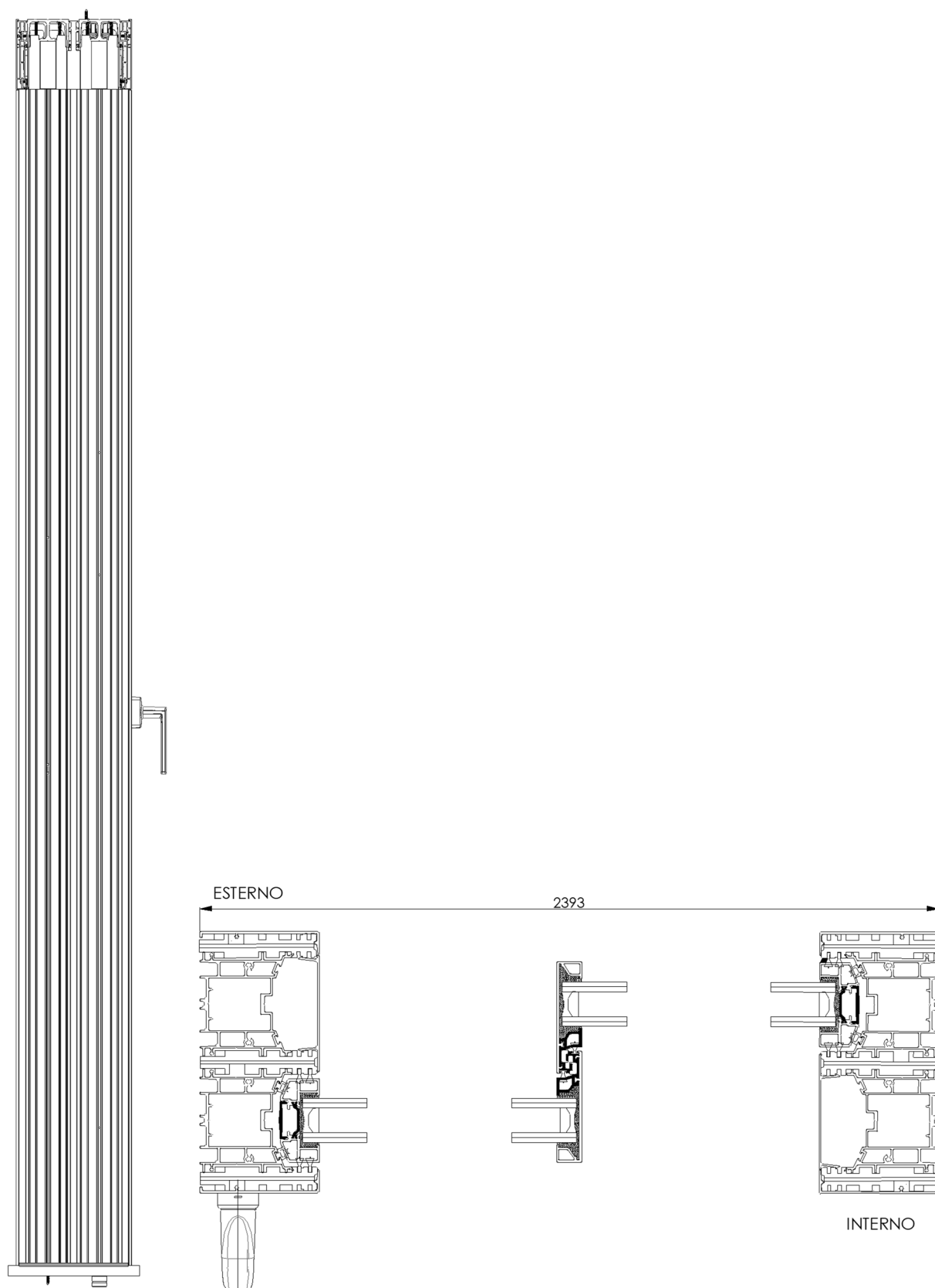
Fig. 2 e Fig. 3. Sezioni verticale ed orizzontale del campione sottoposto a prova (dimensioni nominali dichiarate, espresse in mm)
