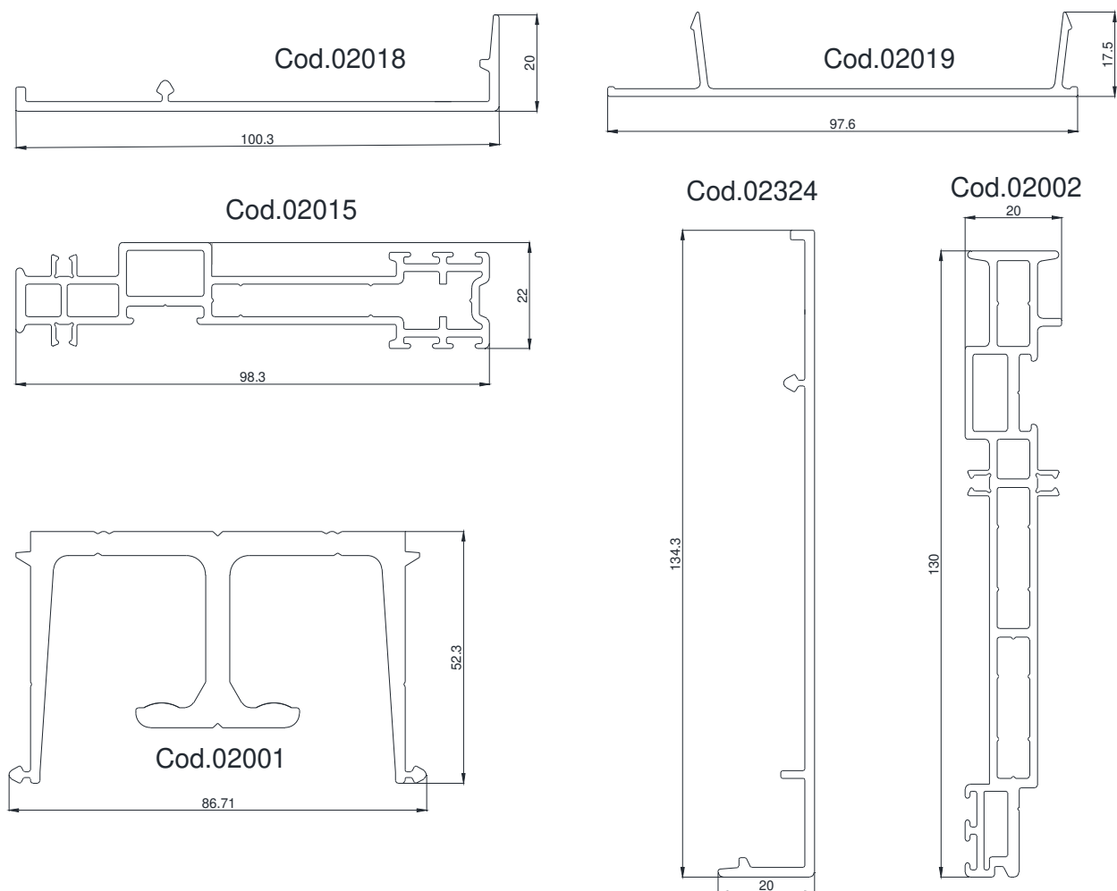
Fig. 7. Distinta dei profili del campione sottoposto a prova (dimensioni nominali dichiarate, espresse in mm)
