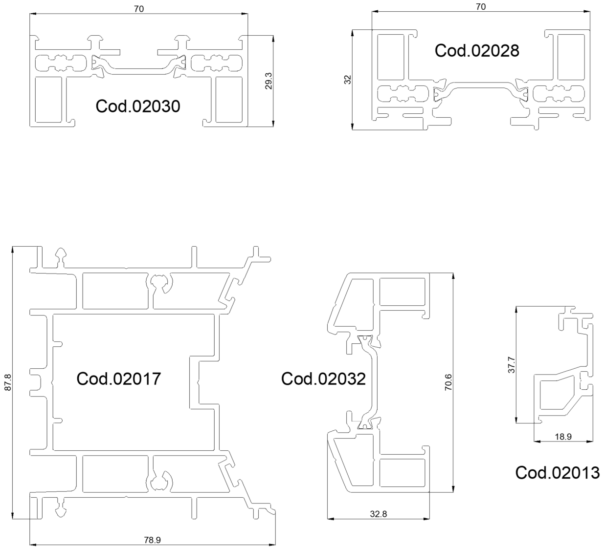
Fig. 6. Distinta dei profili del campione sottoposto a prova (dimensioni nominali dichiarate, espresse in mm)
