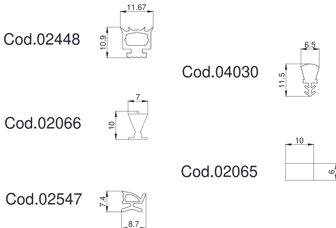
Fig. 9. Distinta delle guarnizioni del campione sottoposto a prova (dimensioni nominali dichiarate, espresse in mm)
