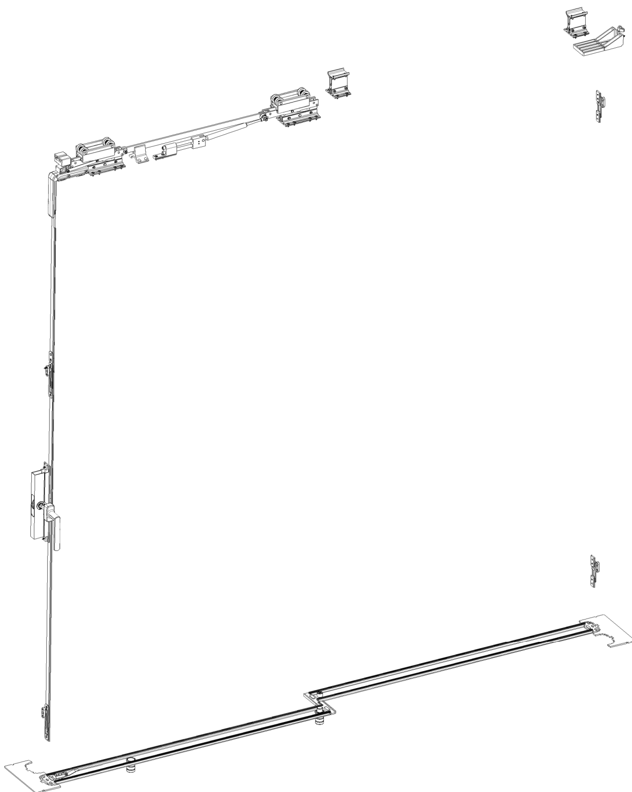
Fig. 4. Vista assometrica degli accessori del campione sottoposto a prova
