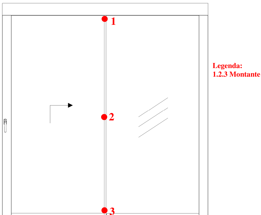
Fig. 10. Assetto sperimentale prova di resistenza al carico del vento vista interna: schema di posizionamento dei trasduttori - posizionati sul lato interno
