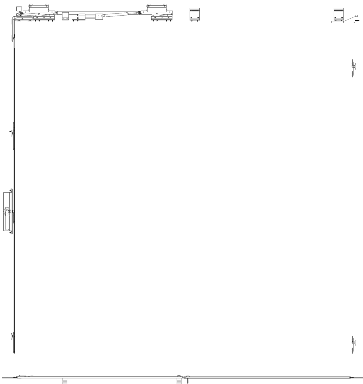
Fig. 5. Posizionamento degli accessori del campione sottoposto a prova
